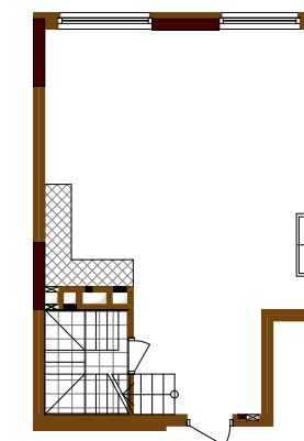
План квартири без перегородок
